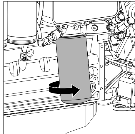
23 Ölfilter montieren
