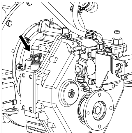
17 Ölstand messen
