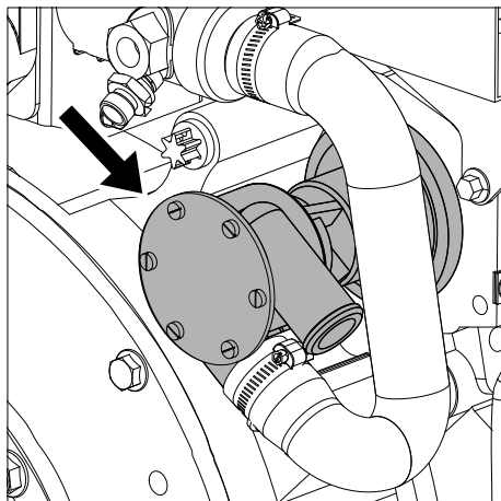
39 Seewasserpumpe kontrollieren
