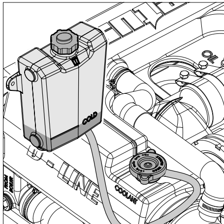
3 Innenwasserkühlsystem
