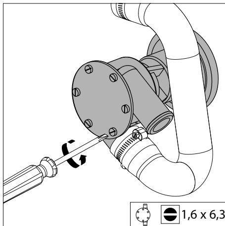
40 Pumpendeckel abmontieren
