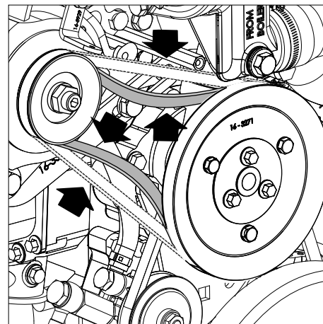
35 Kontrolle Spannung
