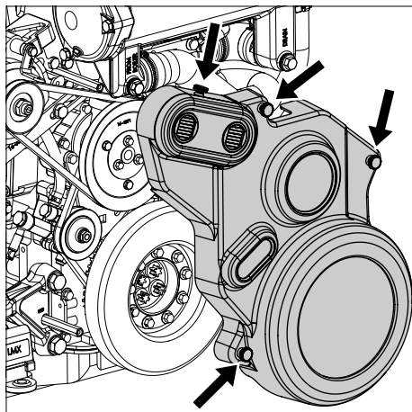
33 Keilriemenabdeckung entfernen
