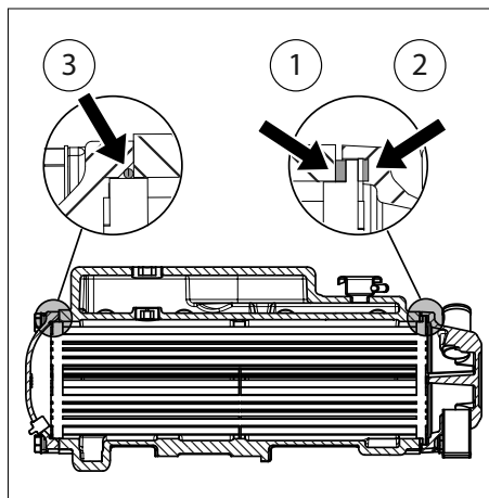
62 Einbau Enddeckel
