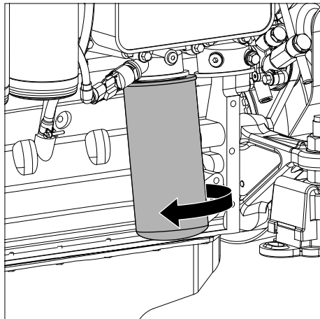
21 Ölfilter abnehmen
