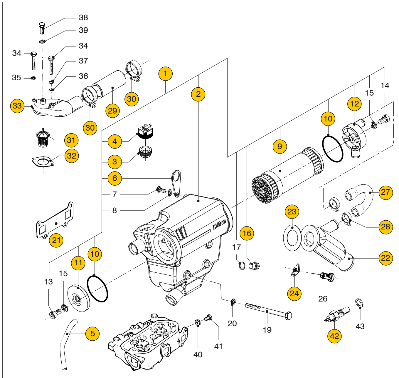
M2.02 M2.04 M2.06 M2.C5 Warmtewisselaar unit 07-2018-> M2.13 M2.18 M2.D5
