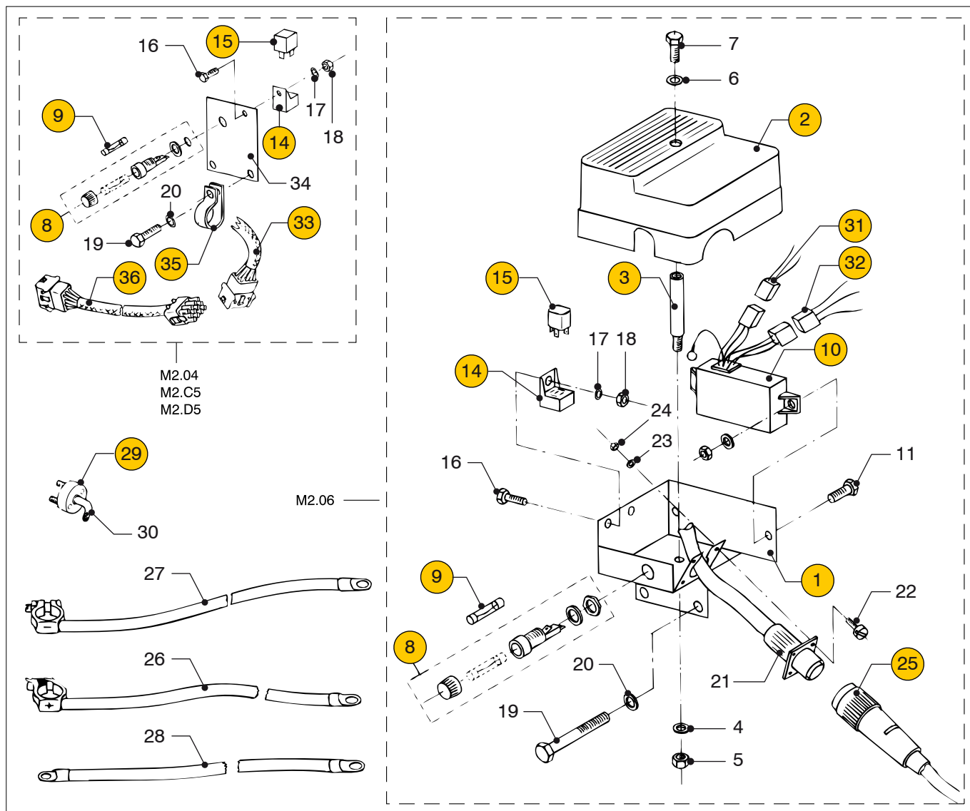
M2.04 M2.06 M2.C5 Bedradingskast, 2001 <- M2.D5
