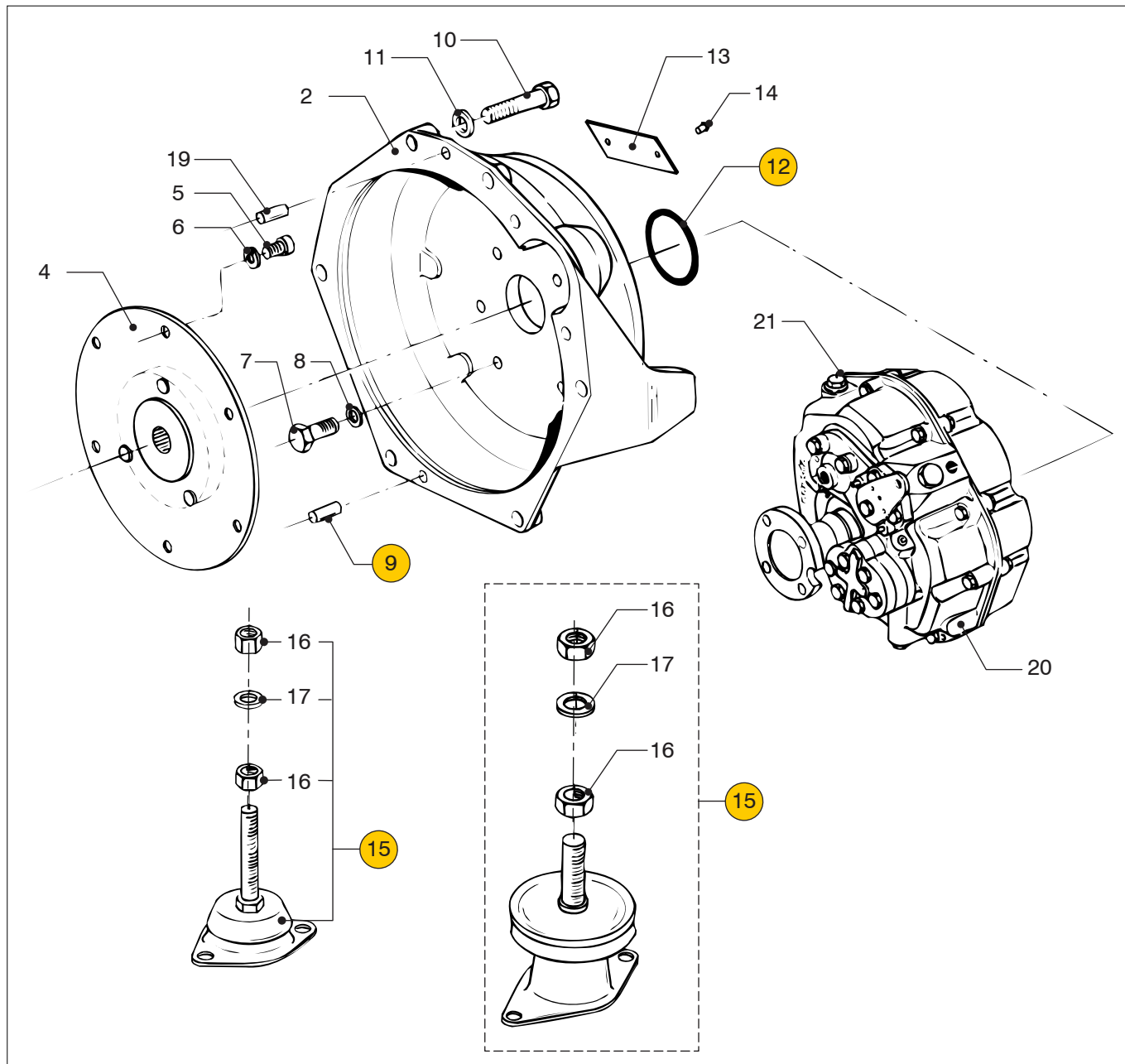
M2.04 M2.06 M2.C5 M2.D5 Vlieg wielhuis PRM
